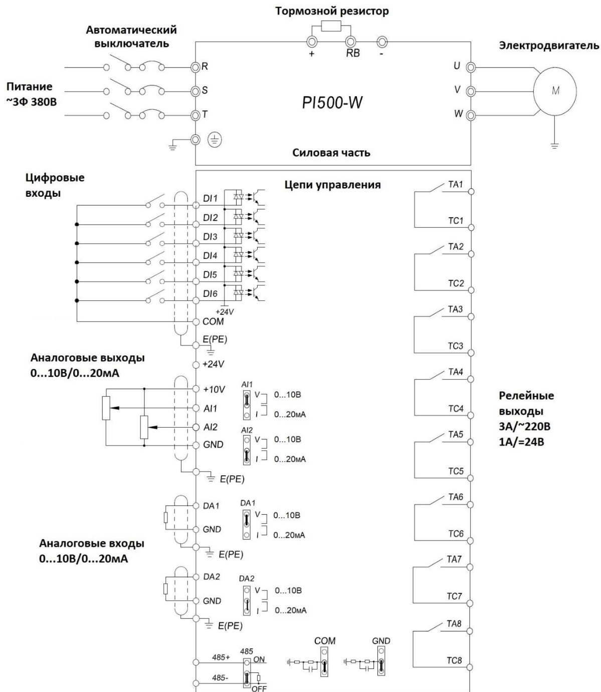
Рисунок 2 – Схема подключений для PI500-W 380В, 18.5 кВт
