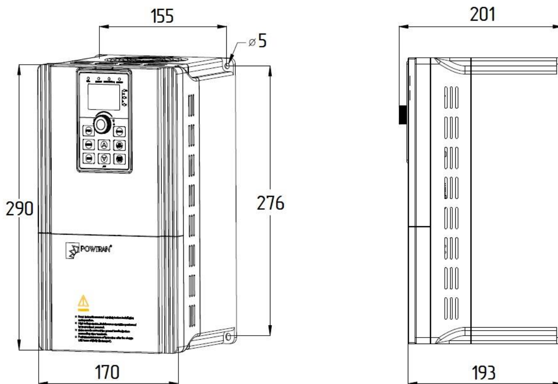
Рисунок 1 – габариты PI500 380В, 18.5 кВт.
